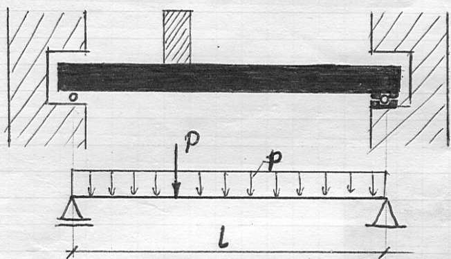
Belka swobodnie podparta
