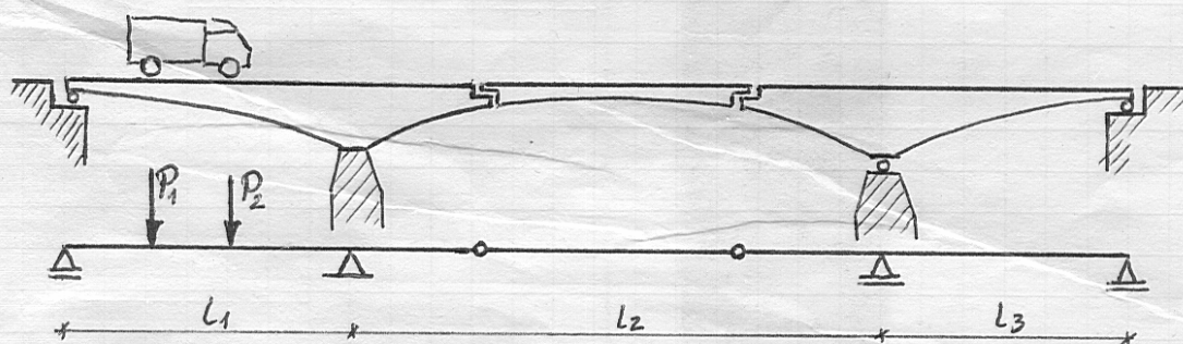
Wspornik
